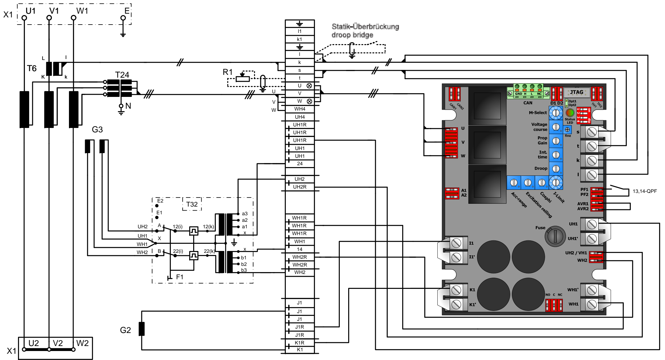
Schaltbild für DIG-Generatoren ( U_N \leq 11,5\text{kV} ) mit Hilfswicklung Connection diagramm for DIG-alternators ( U_N \leq 11,5\text{kV} ) with auxiliary windings
